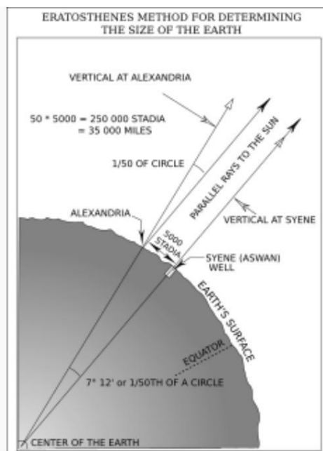
Метод Эратосфена для определения радиуса и окружности Земли.
